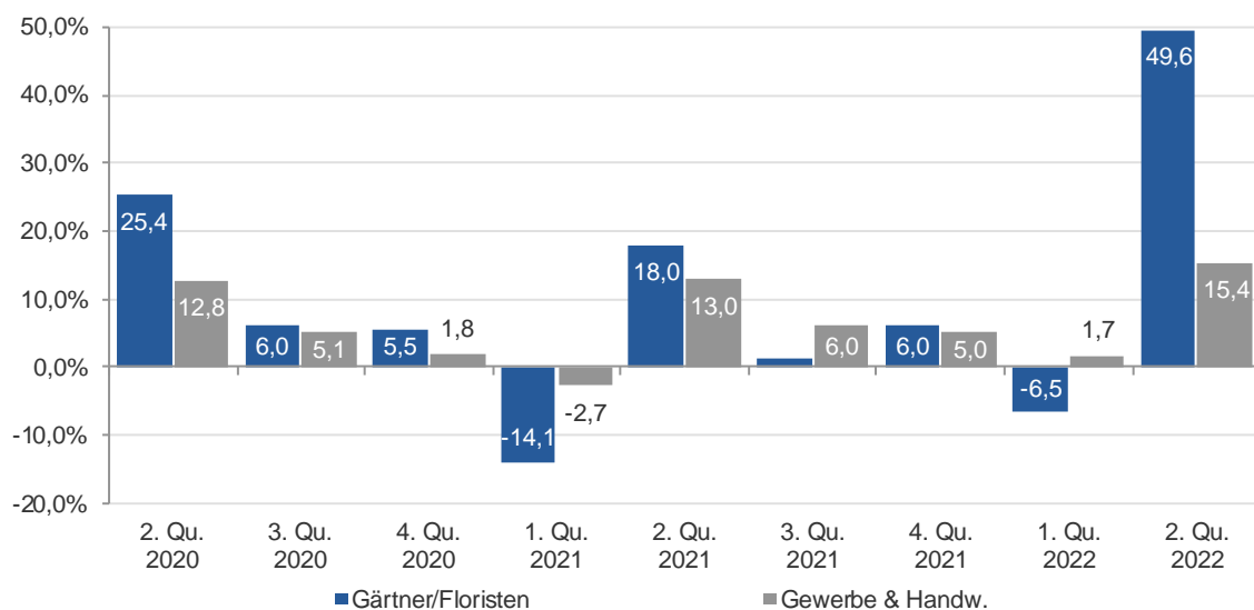
Grafik 9 | Personalbedarf Geplante Veränderung gegenüber dem Vorquartal in Prozent
