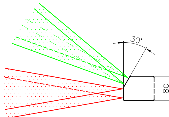
Abb. 3 - Seitenansicht
