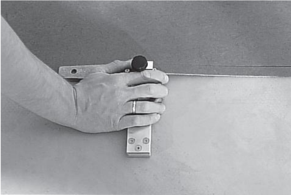
Bild 1 Kantenschnitt
