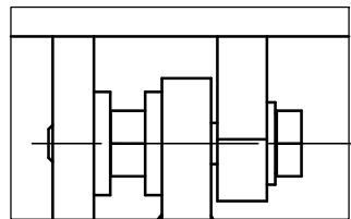
DETAIL B MAßSTAB 1 : 2
