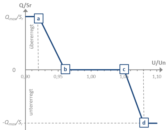
Abbildung 13: Blindleistungs-/Spannungskennlinie Q(U) im Niederspannungsnetz
