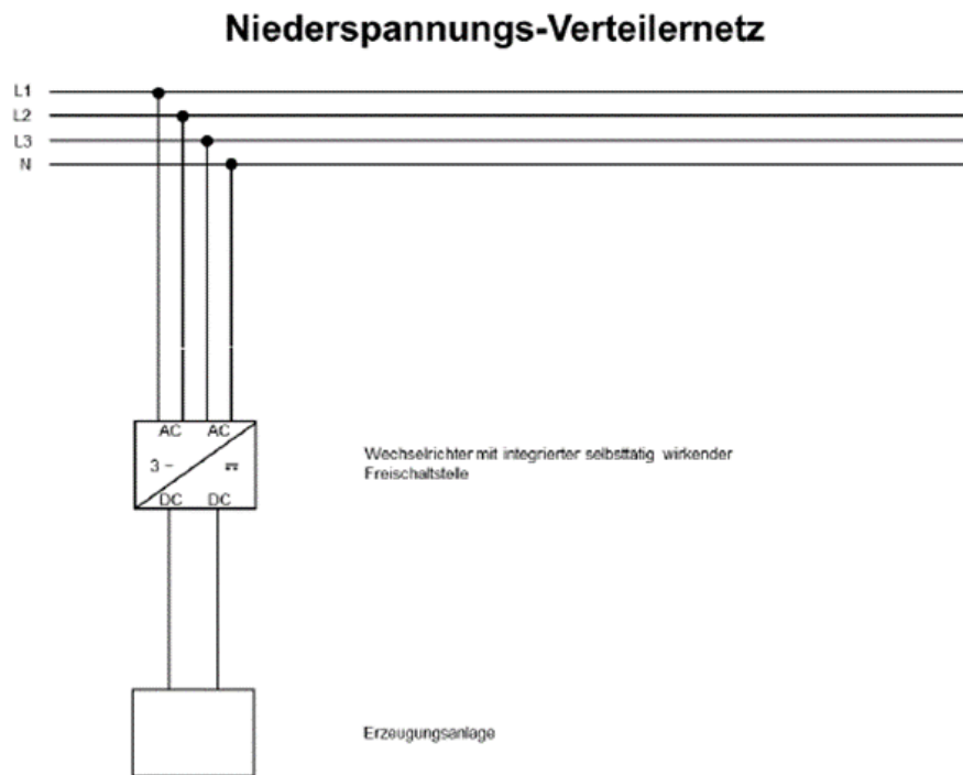
Abbildung 19: Netzanschluss bei Einsatz einer selbsttätig wirkenden Freischnittstelle für mehrphasige Wechselrichter (max. 30 kVA)
