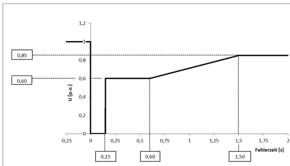
Abbildung 11: FRT-Profil synchrone Stromerzeugungsanlagen
