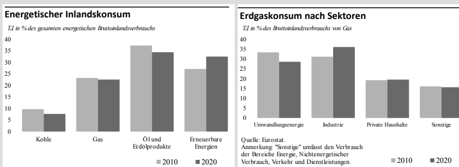
Abbildung 2: Energieverbrauch Österreichs
