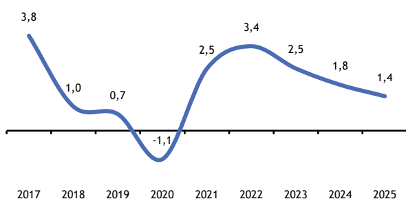
Inflationsrate
