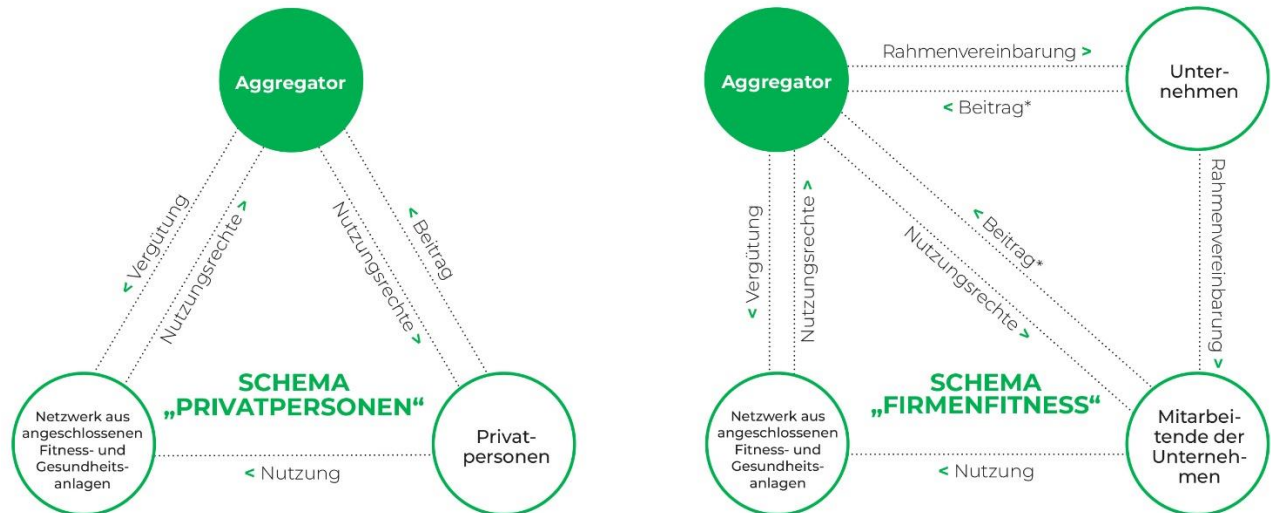
Abb. 12: Aggregatorenmodelle
