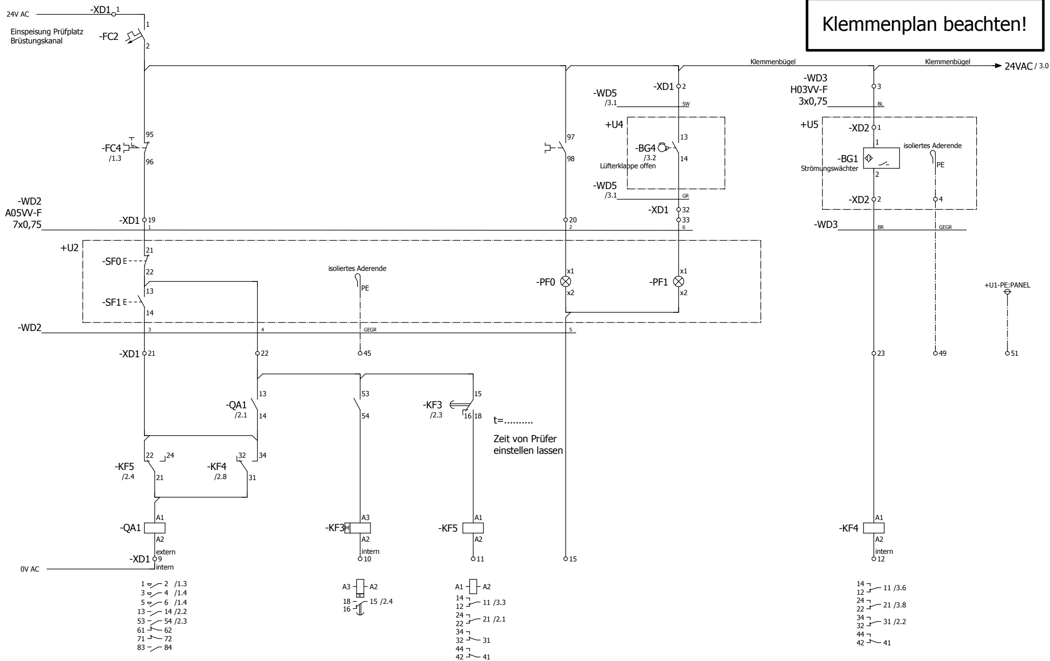
Lüftermotor
