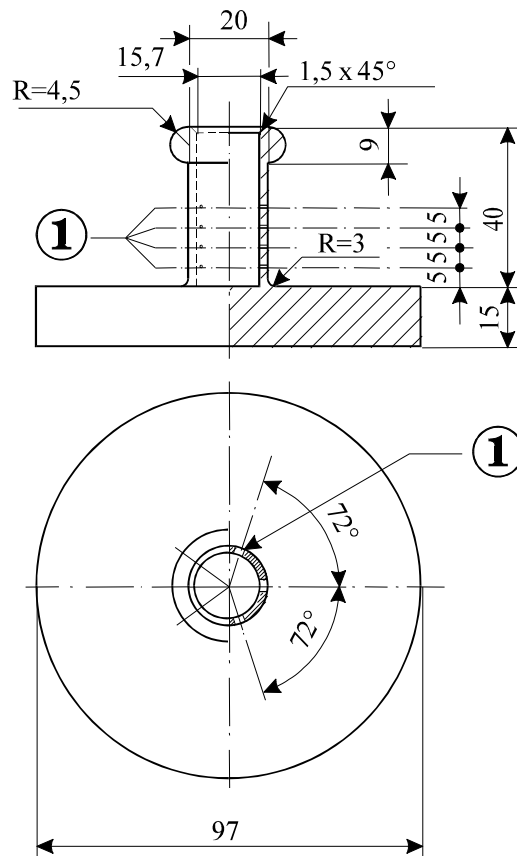
Abb. 3: Hohlter Bronzeyylinder, einseitig verschlossen Aufriss und Grundriss; Masse in mm
