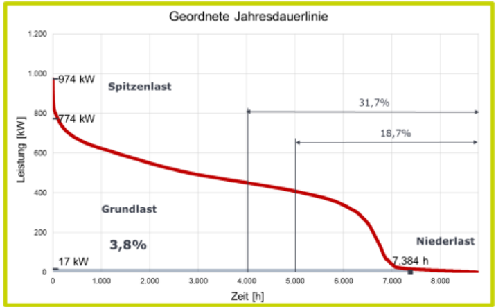
Abbildung 3: Geordnete Jahresdauerlinie
