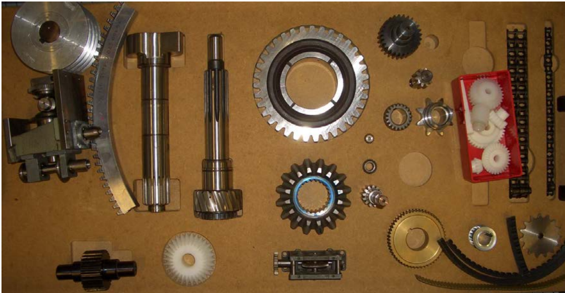
Verzahnung:
