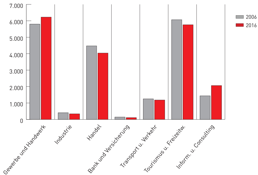
DG-Betriebe Vergleich 2006 - 2016
