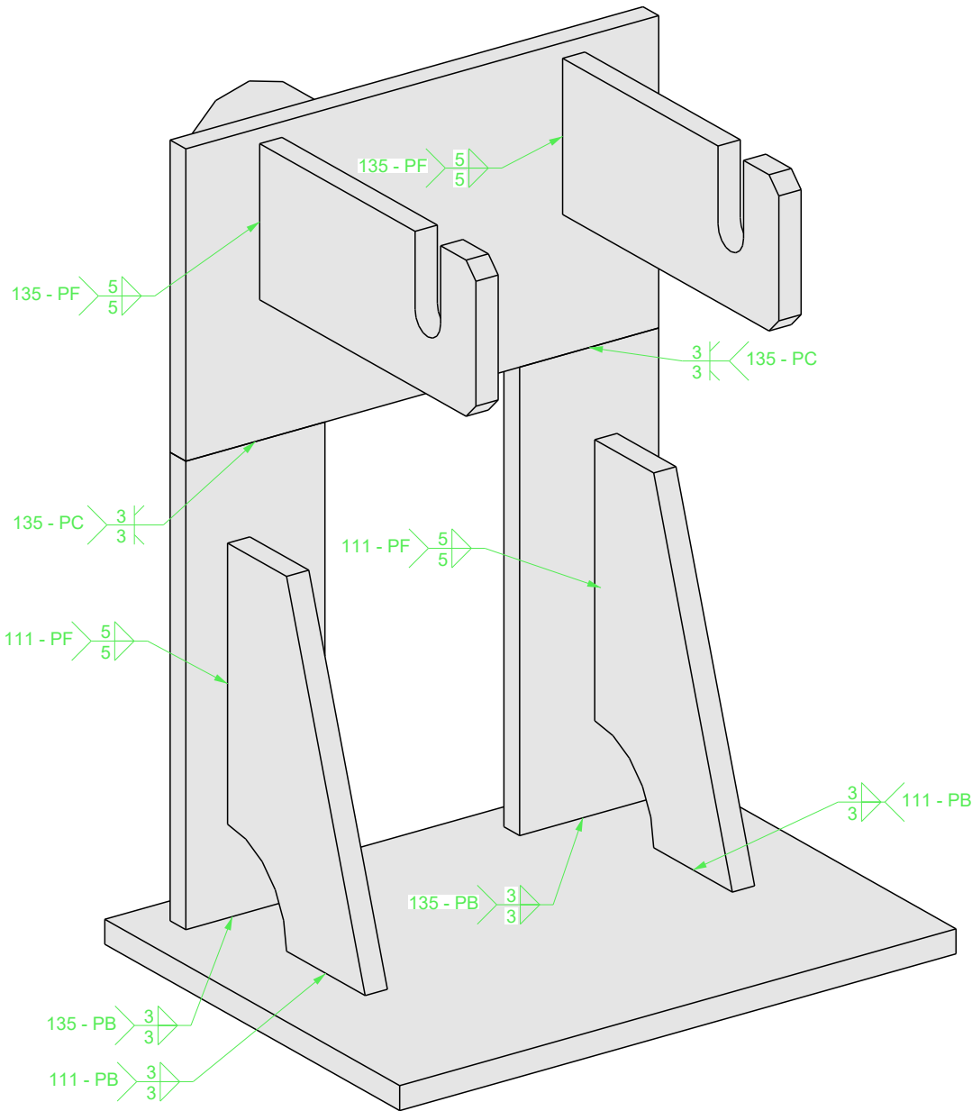
Werkstück Stahl Ansicht vorne
