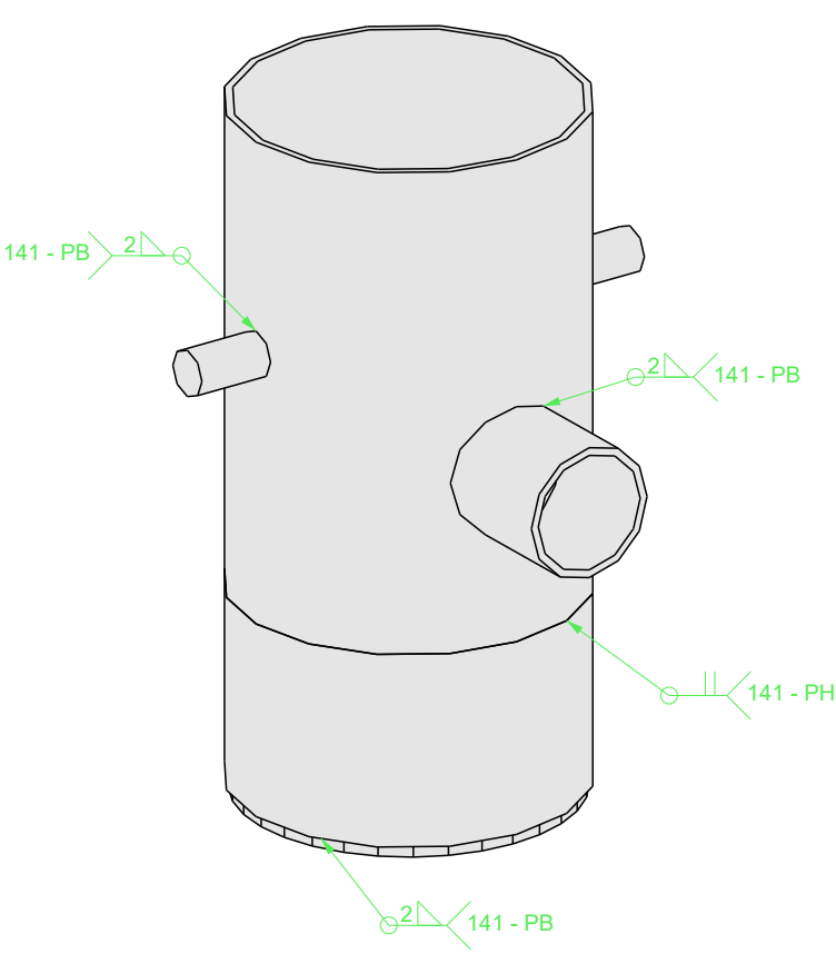
Werkstück Edelstahl Ansicht vorne
