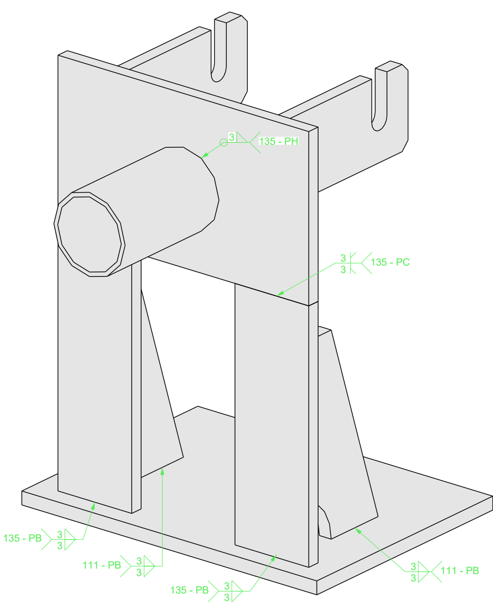
Werkstück Stahl Ansicht hinten
