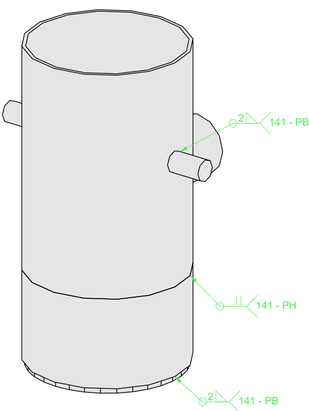
Werkstück Edelstahl Ansicht hinten
