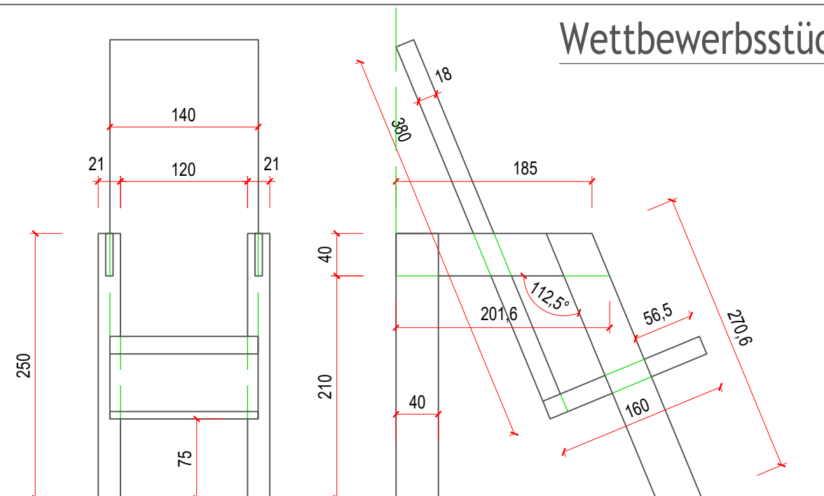
ANSICHTEN M = 1:5
