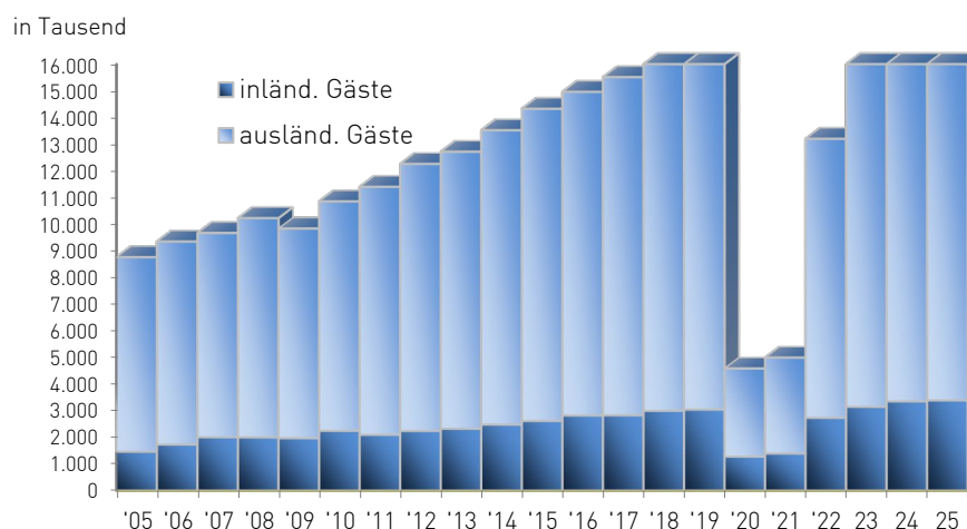
Nächtigungen von In- und Ausländern
